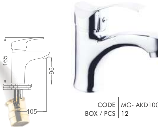
Aqua Beyaz Krom Mix Banyo Bataryası Aqua Mix Bathroom Faucet
