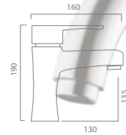
Nil Mix Kuyruklu Eviye Bataryası Nil Mix With Tail Sink Kitchen Faucet
