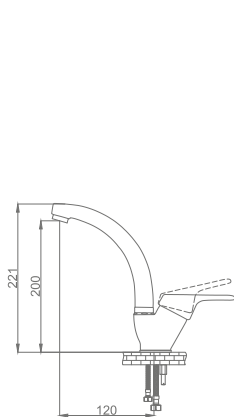
Mega Mix Kuğu Lavabo Bataryası Mega Mix Swan Rotating Sink Faucet
