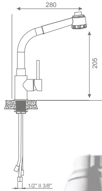
Life Villa Eviye Bataryası Life Villa Sink Faucet
