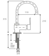
Truva Mix Kugu Eviye Bataryası Truva Mix Swan Kitchen Faucet
