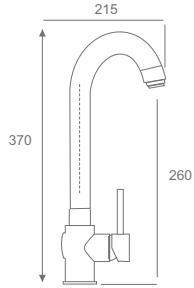
Life Max Spiralli Eviye Bataryası Life Max Spiralli Sink Faucet
