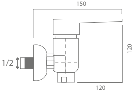
Nil Mix Lavabo Bataryası Nil Mix Basin Faucet
