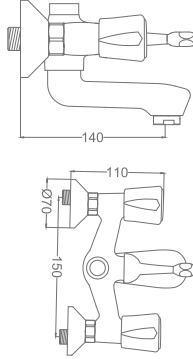
Nida Klasik Kuğu Kuyruklu Eviye Bataryası Nida Classic Swan Neck Kitchen Faucet
