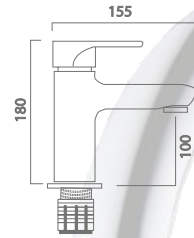
Snow Mix Kuyruklu Kuğu Lavabo Bataryası Snow Mix With Tail Swan Rotating Sink Faucet
