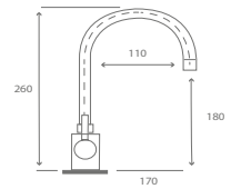
Ege Mix Eviye Bataryası Akordion Ege Mix Sink Faucet
