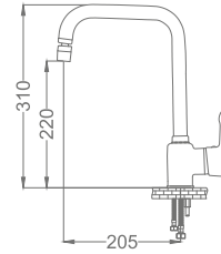
Zümrüt Mix Siyah Krom Banyo Bataryası Zümrüt Mix Bathroom Faucet
