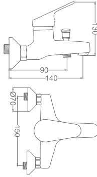
Mega Mix Kuğu Eviye Bataryası Mega Mix Swan Kitchen Faucet
