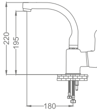
Zümrüt Mix Siyah Altın Banyo Bataryası Zümrüt Mix Bathroom Faucet
