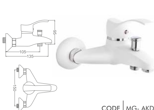
Aqua Beyaz Krom Mix Banyo Bataryası Aqua Mix Bathroom Faucet
