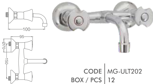
Düden Klasik Kuğu Borulu Eviye Bataryası Düden Classic Kitchen Faucet with Swan Spout
