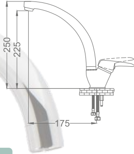
Karya Mix Baston Kuğu eviye bataryası Karya Mix Swan Neck Kitchen Faucet
