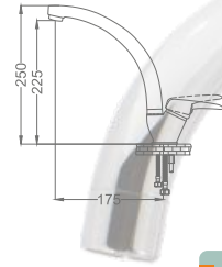
Karya Mix Yüksek Type Lavabo bataryası Karya Mix Basın Faucet
