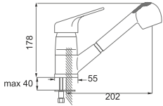
Mercan Mix Bide Bataryası Mercan Mix Bidet Tap Mixer
