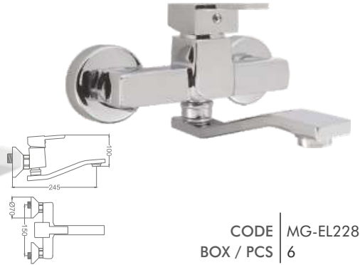
Milenyum Mix Perlatörlü Lavabo Bataryası Milenyum Mix Basin Faucet
