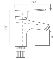
Ege Mix Kuyruklu Kuğu Lavabo Bataryası Ege Mix With Tail Swan Rotating Sink Faucet
