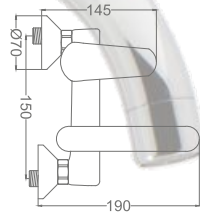
Kale Mix Eviye Bataryası Kale Mix Kitchen Faucet
