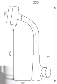
Mega Mix Spiralli Eviye Bataryası Mega Spiralli Sink Faucet
