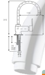
Mix Truva Mix Kuyruklu Kuğu Lavabo Bataryası Truva Mix With Tail Swan Rotating Sink Faucet
