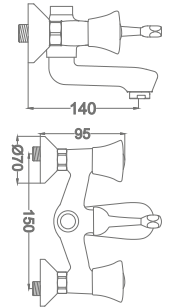
Düden Klasik Eviye Bataryası Düden Classic Kitchen Faucet
