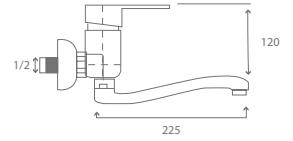
Ege Mix Kuğu Lavabo Bataryası Ege Mix Swan Rotating Sink Faucet
