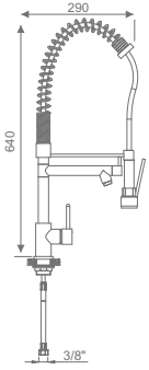
Life Arıtmalı Eviye Bataryası Life Purificatiom Sink Faucet
