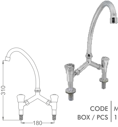
Mega Klasik Köprülü Lavabo Batayısı Mega Classic Bridge Basin Faucet
