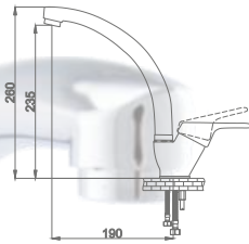
Efes Mix Lavabo Bataryası Efes Mix Basin Mixer
