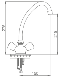
Mega Klasik Dönerli Lavabo Batayısı Mega Classic Bathroom Faucet
