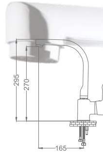
Mira Mix Kuğu Lavabo Bataryası Mira Mix Swan Neck Kitchen Faucet
