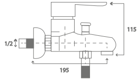
Nil Mix Aplike Eviye Bataryası Nil Mix Ornamented Kitchen Faucet
