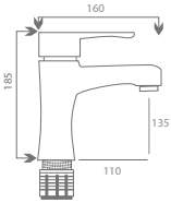
Truva Mix Üsten Aplike Eviye Bataryası- Kuyruklu Truva Mix Front Type Applique Sink Faucet
