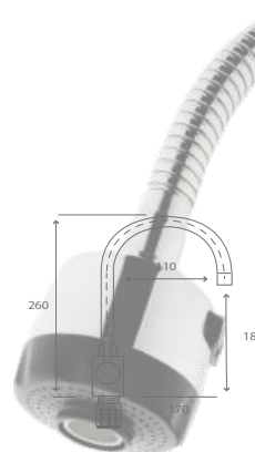
Ege Mix Kuyruklu Kuğu Lavabo Bataryası Ege Mix With Tail Swan Rotating Sink Faucet
