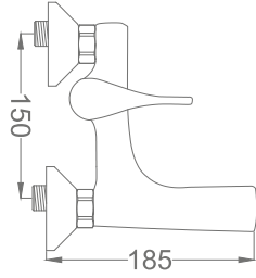
Platin Eviye Bataryası Platin Kitchen Faucet
