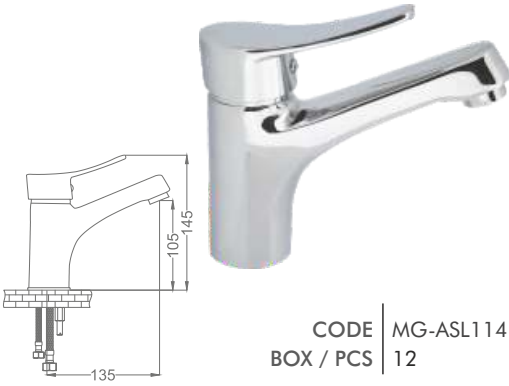
Efes Mix Eviye Bataryası Efes Mix Kitchen Faucet
