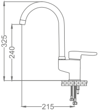
Asos Mix Kugu Eviye Bataryası Asos Mix Swan Kitchen Faucet
