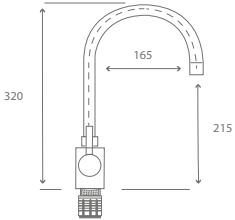
Ege Mix Köşeli Eviye Bataryası Ege Mix Sink Faucet
