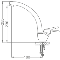
DeltaMix Kuğu Lavabo Bataryası Delta Mix Swan Sink Faucet
