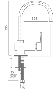
Nil Mix Kuyruklu Lavabo Bataryası Nil Mix With Tail Basin Faucet
