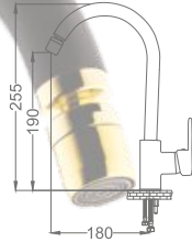
City Mix Kuğu Lavabo Bataryası City Mix Swan Rotating Sink Faucet
