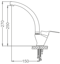
Smart Mix Kuğu Lavabo Bataryası Smart Mix Swan Rotating Sink Faucet
