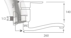
Nil Mix Kuğu Lavabo Bataryası Nil Mix Swan Neck Kitchen Faucet
