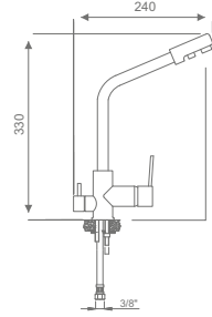
Life Vega Spiralli Eviye Bataryası Life Vega Spiralli Sink Faucet
