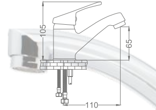
Delta Mix Yüksek Tip Lavabo Bataryası Delta Mix Basin Faucet
