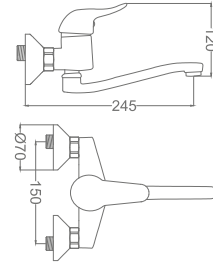
Mercan Mix Eviye Bataryası Mercan Mix Kitchen Faucet
