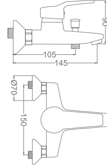
Smart Mix Banyo Bataryası Smart Mix Bathroom Faucet
