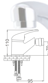
Ocean Mix Taharet Bataryası Ocean Lavatory Faucet
