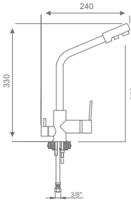
Life Ultra Spiralli Eviye Bataryası Life Ultra Spiralli Sink Faucet
