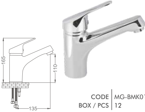
Mega Mix Eviye Bataryası Mega Mix Kitchen Faucet
