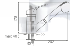
Efes Mix Bide Bataryası Efes Mix Bidet Tap Mixer
