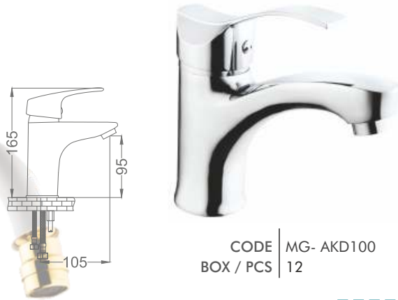
Aqua Mix Lavabo Bataryası Aqua Mix Basin Faucet
