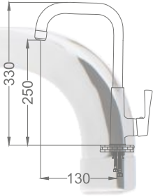
Platin Lavabo Bataryası Platin Basin Faucet
