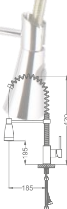
Endüstrüyel Eviye Bataryası Industrial Kitchen Faucet
