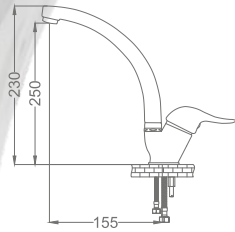
Mercan Mix Yüksek Tip Lavabo Bataryası Mercan Mix High Type Faucet
