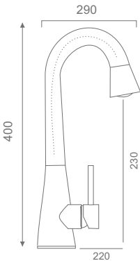
Life Ultra Spiralli Eviye Bataryası Life Ultra Spiralli Sink Faucet
