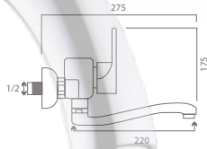
Truva Mix Önden Aplike Eviye Bataryası- Kuyruklu Truva Mix Front Type Applique Sink Faucet
