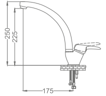
Line Mix Kuğu Eviye Bataryası Line Mix Swan Rotating Sink Faucet
