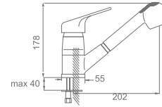
Kale Mix Kuğu Evye Bataryası Kale Mix Swan Neck Kitchen Faucet
