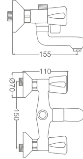
İris Klasik Dönerli Lavabo Bataryası Iris Classic Rotating Sink Faucet
