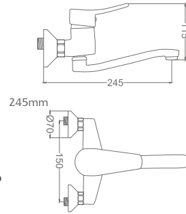
Efes Mix Spiralli Eviye Bataryası Efes Mix Spiral Kitchen Faucet
